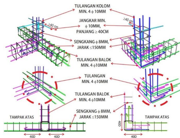
Gambar 8. Bentuk Hubungan Kolom-Balok Sloof dan Fondasi Batu Kali Yang Disarankan Untuk Bangunan Tahan Gempa (Sumber: Boen (2010))
