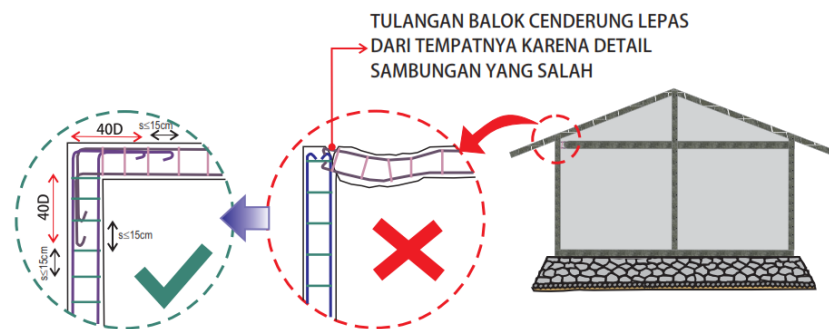
Gambar 5. Bentuk Hubungan Balok-Kolom Yang Disarankan Untuk Bangunan Tahan Gempa (Sumber: Boen (2010))
