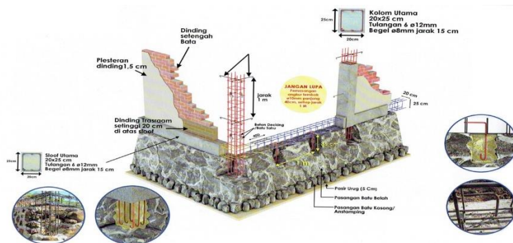
Gambar 7. Tipikal Bentuk Sambungan Kolom-Balok Sloof dan Fondasu Batu Kali Yang Disarankan Untuk Bangunan Tahan Gempa ( https://teddyboen.com/publications.html )
