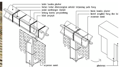
Gambar 8. Perakitan Kolom-Balok
