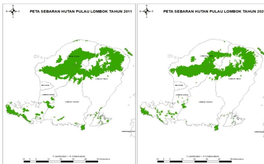
Gambar 2. Perubahan bentuk sebaran hutan akibat deforestasi di pulau Lombok (Sumber : peta penutupan lahan Planologi Kehutanan).
