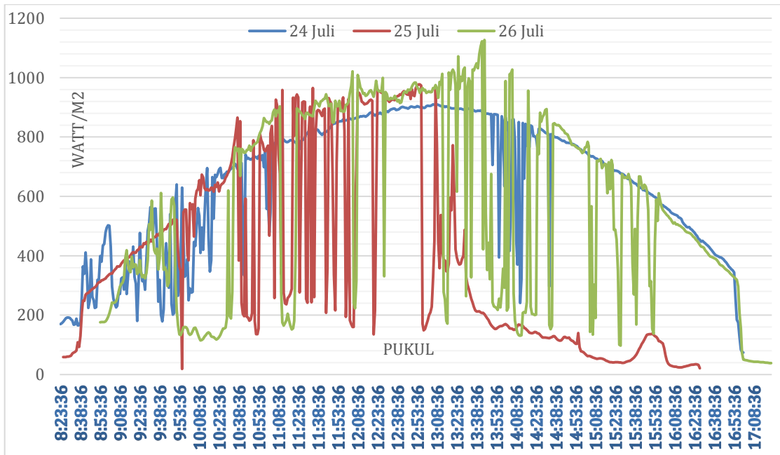
Gambar 4 Grafik Pengukuran Intensitas Matahari (Watt/m 2 ) menggunakan SPM Lutron pada tgl. 24, 25 dan 26 Juli 2023
