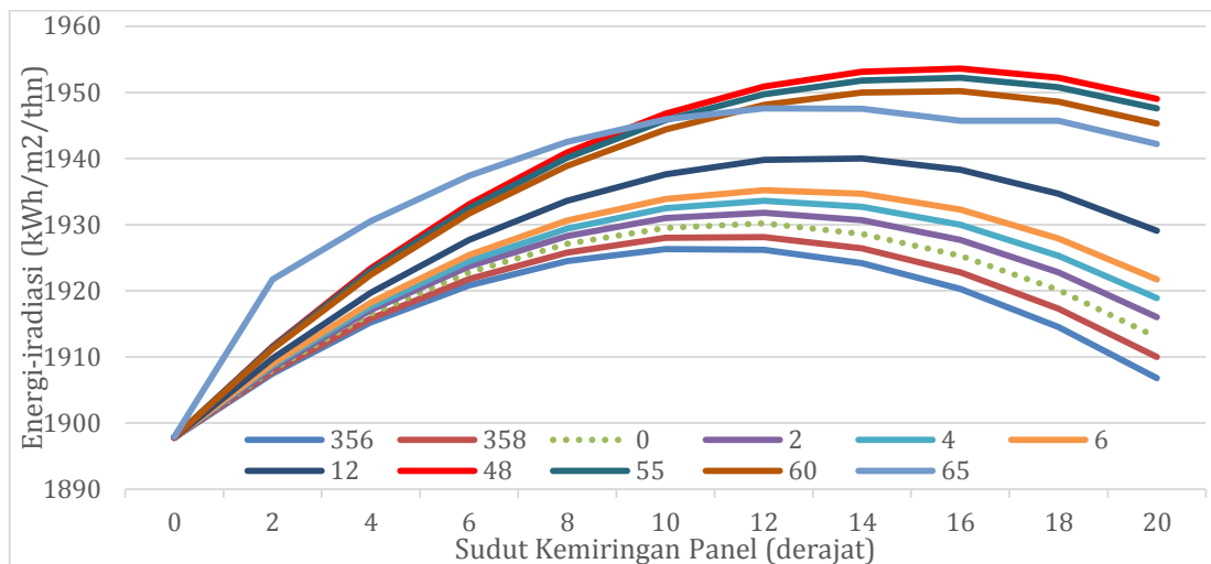
Gambar 5 Grafik Hubungan Iradiasi Sinar Matahari terhadap Sudut Kemiringan pada Tiap Sudut Azimut Berbeda Menggunakan Global Solar Atlas
